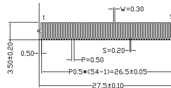
DETAIL B 2:1
